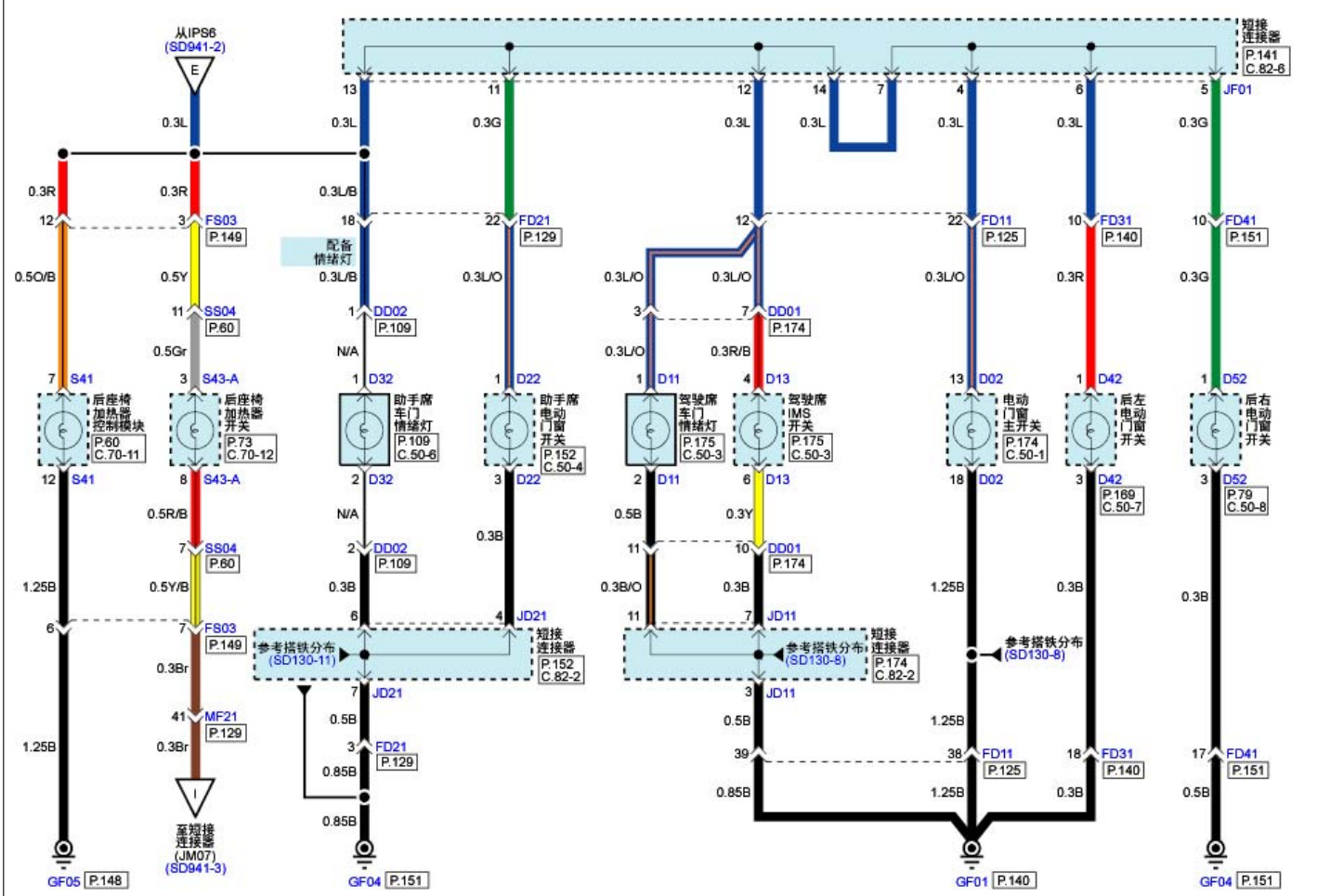
照明灯(4)
